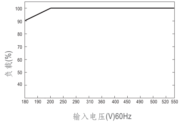
■ 态特性曲线
