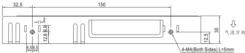
端子Pin脚分步
